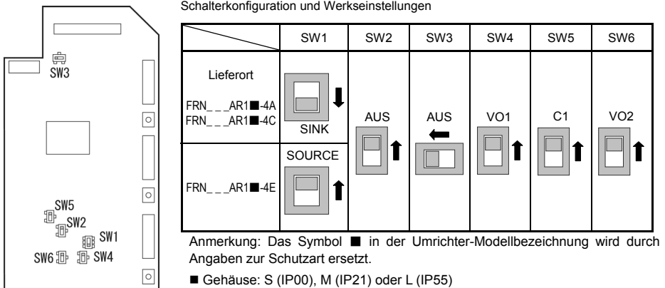
Abbildung 2.9 Anordnung der Schiebeschalter auf der Steuerungsplatine
